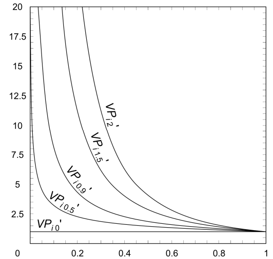
Abb. 3b: Erste Ableitungen VP_{ii}' zu Abb. 3a
