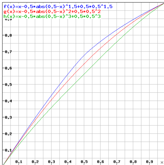
Abb. 4a: Egalitaristische Funktionen VE_{VARS1,5} , 2 , 3
